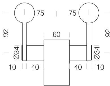
4R Fin Divider Rail ®
