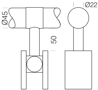
4E Inline Stem Toprail
