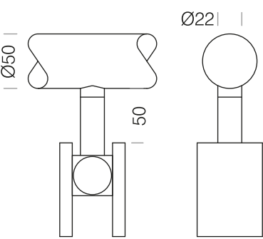
4E Inline Stem Toprail
