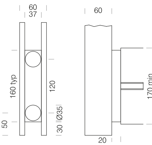
6G Fin Side Fixing
