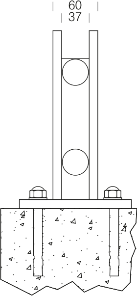
6F Top Fixing
