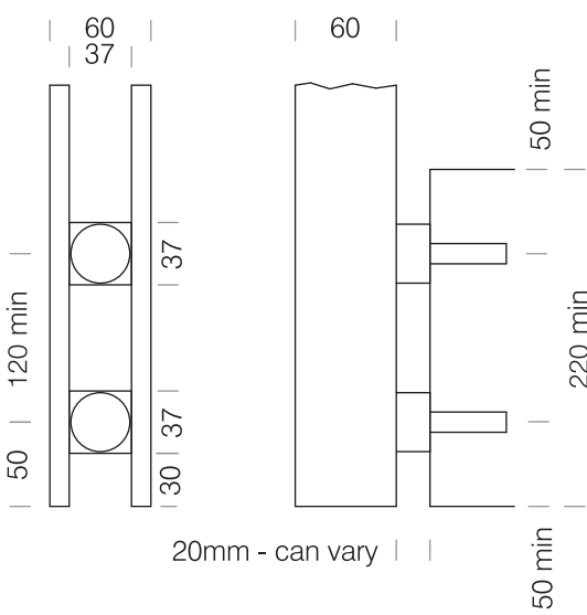
6E Side Fixing
